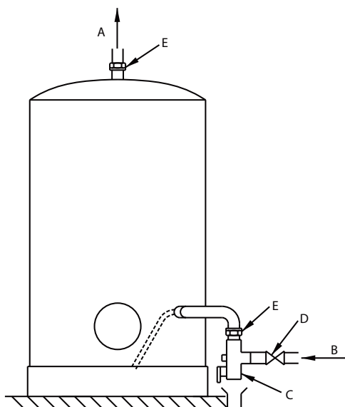
Figura 12 - Modello pavimento su anello
