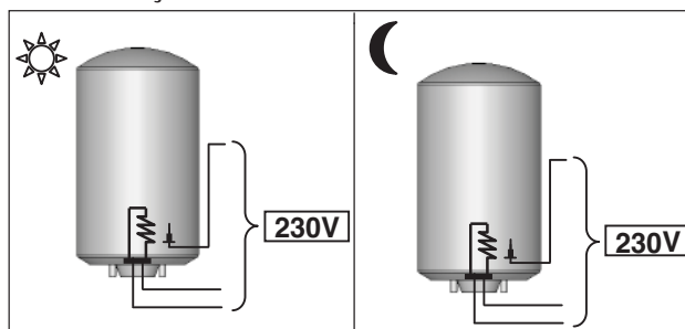
Figura 14 – PROfessional TECH Alimentaçãu permanente
