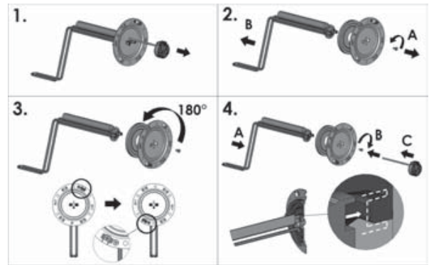
Figura 8 - Montaggio della resistenza modello HORD in configurazione "Sinistra" (vedere Libretto 2.2 figura 8)
