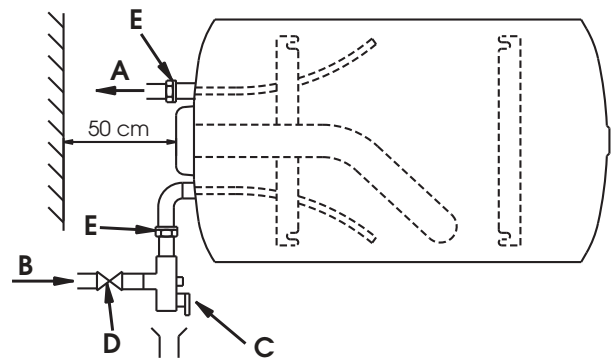
Figura 9 - Modello orizzontale sull'elemento di protezione - tubi di alimentazione a sinistra
