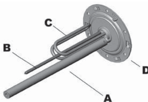
Figura 1 - Resistência a imersão + ânodo de magnésio
