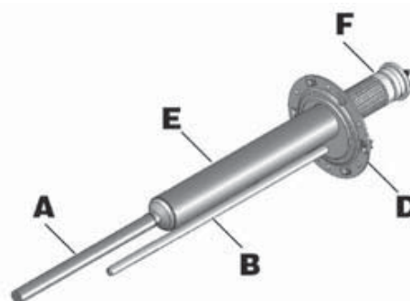
Figura 2 - Resistência esteatite + ânodo de magnésio
