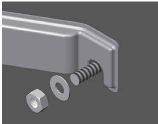
Figura 5 - Montagem presilha de fixação
