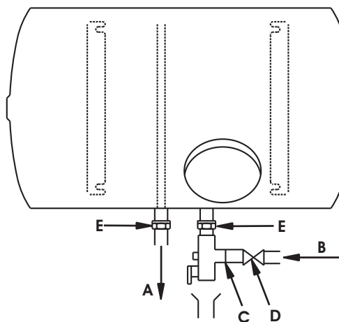
Figura 10 - Modelo horizontal em casquilho
