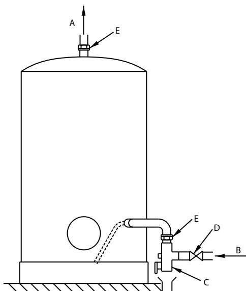
Figura 12 - Modelo sobre em casquilho
