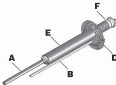
Figura 2 - Resistenza steatite + anodo di magnesio
