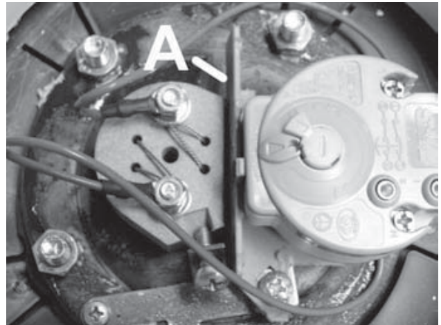
Figura 17 – Separatore plastico / A : separatore plastico
