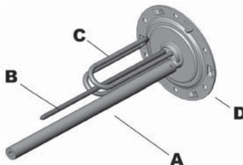
Figura 1 - Resistenza a immersione + anodo di magnesio
