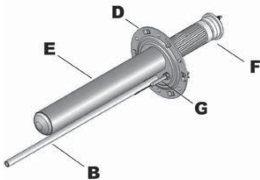
Figura 3 - Resistência esteatite + ânodo PROfessional TECH
