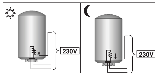
Figura 14 – Professional Tech alimentazione permanente
