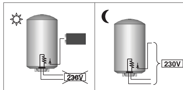
Figura 13 – Professional Tech alimentazione notturna + batterie
