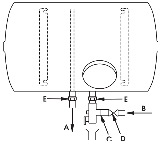
Figura 10 - Modello orizzontale su ghiera
