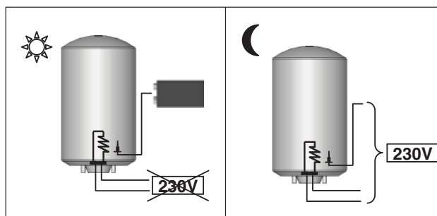
Figura 13 – PROfessional TECH Alimentaçãu nocturna + baterias
