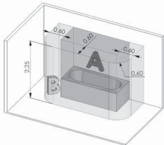
Figura 4 - Zona di installazione / A : Volume involucro / B : Volume di protezione
